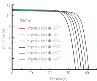
Curva de corriente - tensión (LR4-60HPH-365M)
