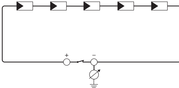
Imagen 13: Representación esquemática de la medición
