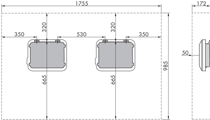
Imagen 7: Distancias recomendadas (Medidas en mm)
