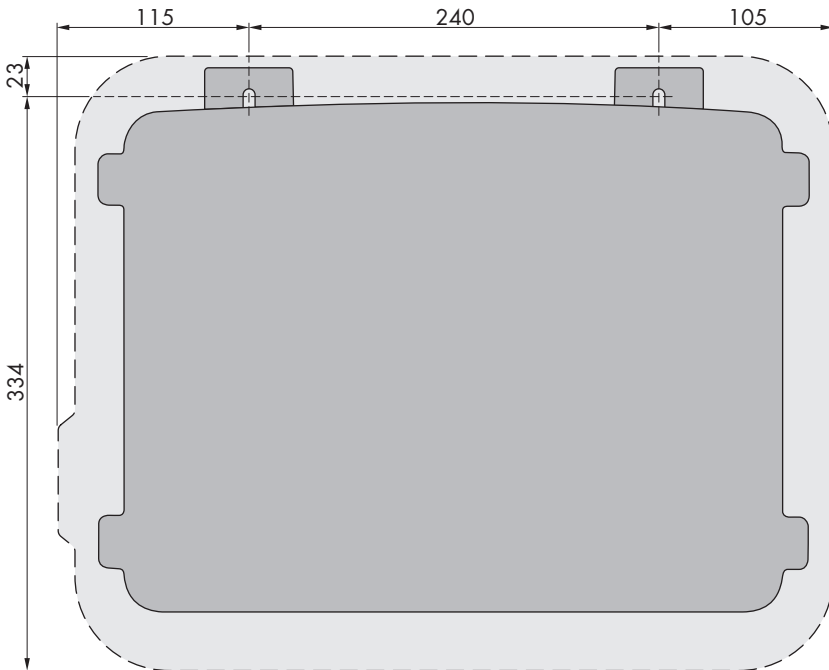
Imagen 6: Posición de los puntos de fijación (Medidas en mm)
