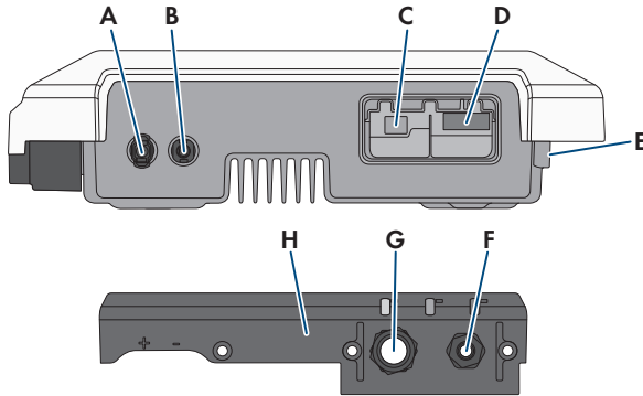
Imagen 8: Áreas de conexión y aberturas en la carcasa en la parte inferior del inversor
